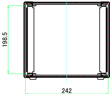
B-B ( 1 : 5.5 )
