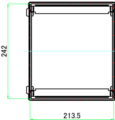
A-A ( 1 : 5.5 )
