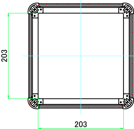
C-C ( 1 : 5.5 )
